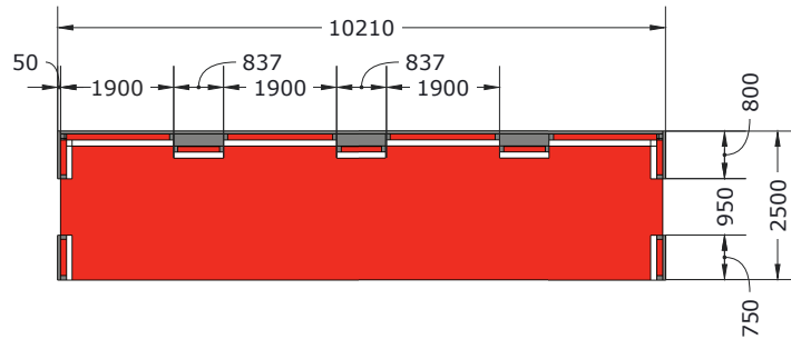
Schnitt B-B
