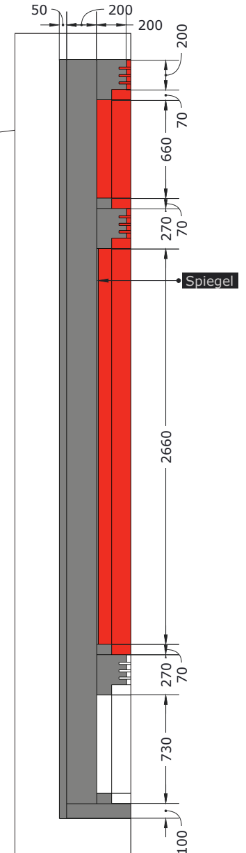
Detail: Wandprofil M 1:25
