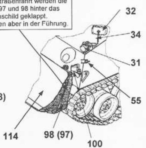
Bergen von einem Fahrzeug mit der Hauptwinde
