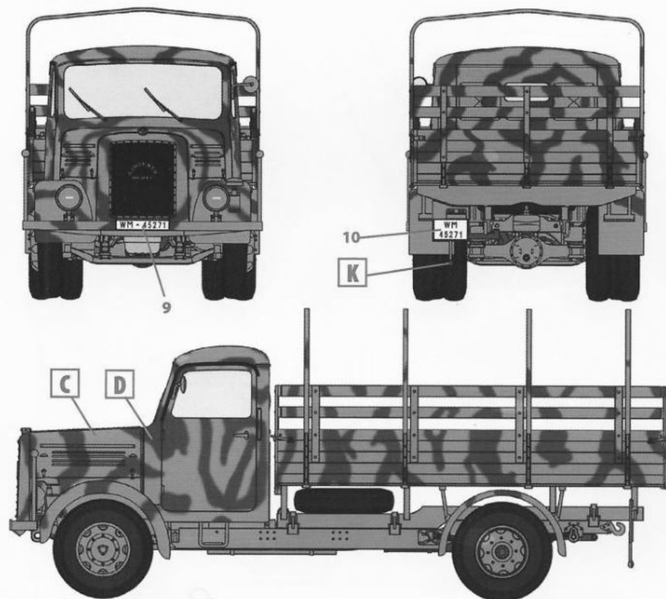
4. KHD S3000, Франция, лето 1944 г. KHD S3000, France, Summer 1944
