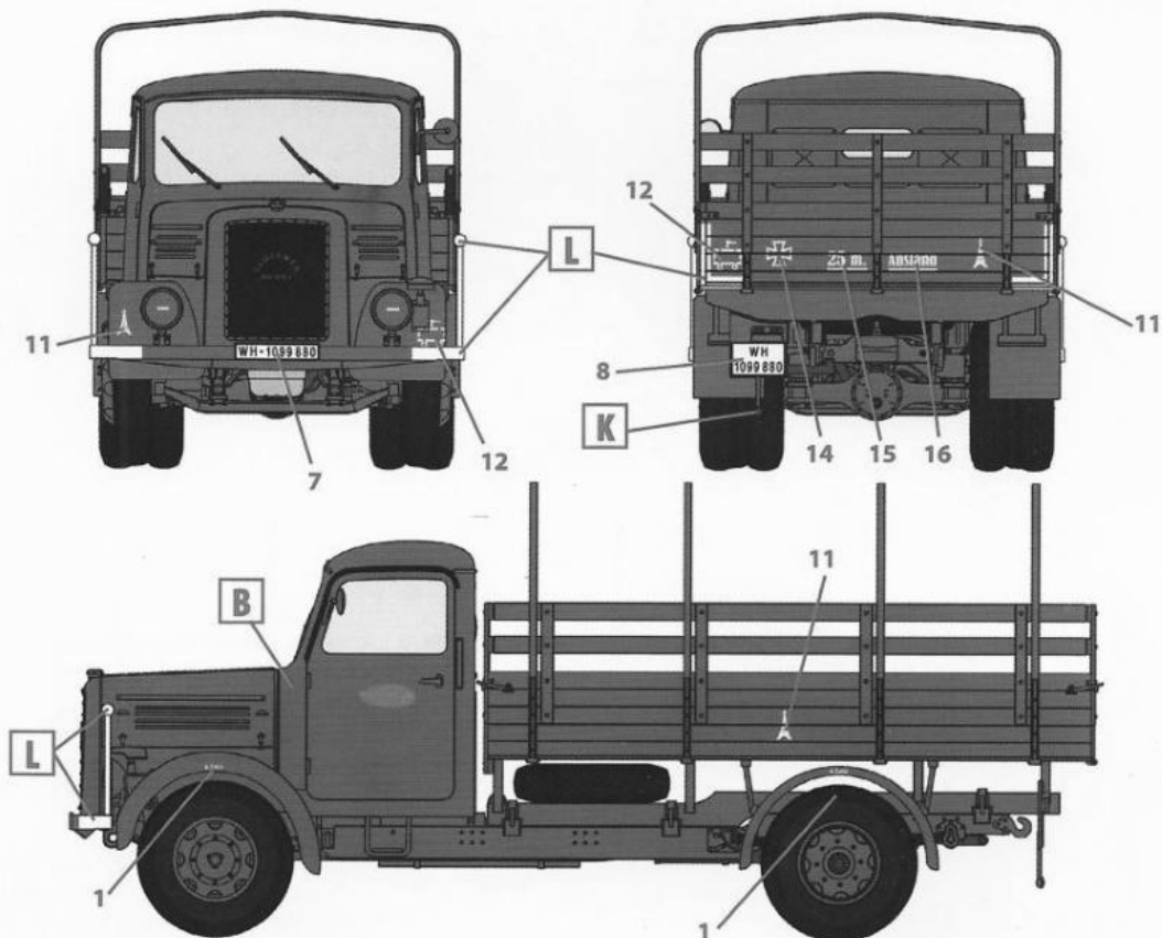
3. KHD S3000, 23-я ТД, Украина, лето 1942 г. KHD S3000, 23d PzD, Ukraine, Summer 1942
