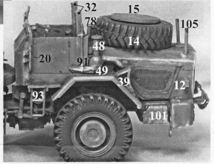
Tankstutzen (78) kann wahlweise durch das Tarnnetz (72) ersetzt werden. Filler neck (78) could be exchanged by camouflage net (72).
