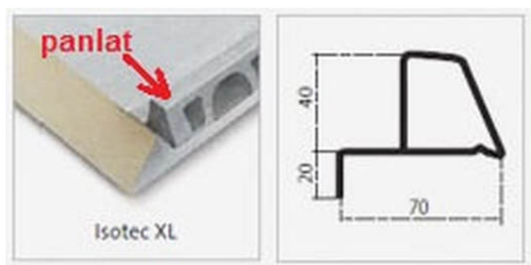
afb. 15.4.1 - 2 De panlat van het Isotec sarking element
