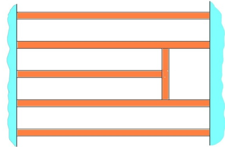
afb.08.3.1 - 3 Balklaag met uitwisseling (raveling)
