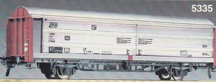
5335 · Gedeckter Schiebewandwagen, Modell des Hbis 299 der DB, LüP: 161 mm. Silber/rotbraune DB-Lackierung, vorbildentsprechend beschriftet, Seitenwände zum Öffnen und Schließen.
