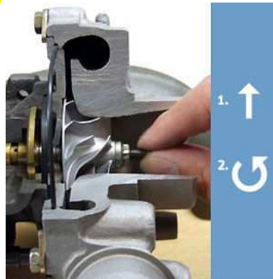
Bild 4 Zum Prüfen der Lagerung wird die Läuferwelle an der Mutter des Verdichterrads leicht angehoben (1). Beim Drehen (2) der Welle darf kein Schleifgeräusch zu hören oder Druckwiderstand feststellbar sein.
