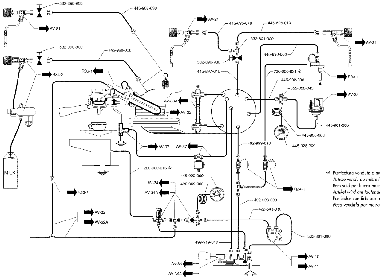
INSTALACION HIDRAULICA SISTEMA HIDRÁULICO
