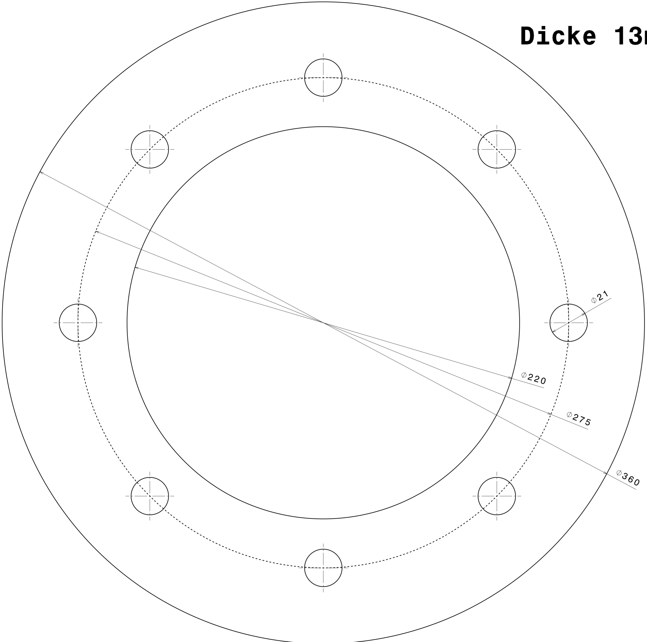
Vorderansicht Maßstab: 1:1
