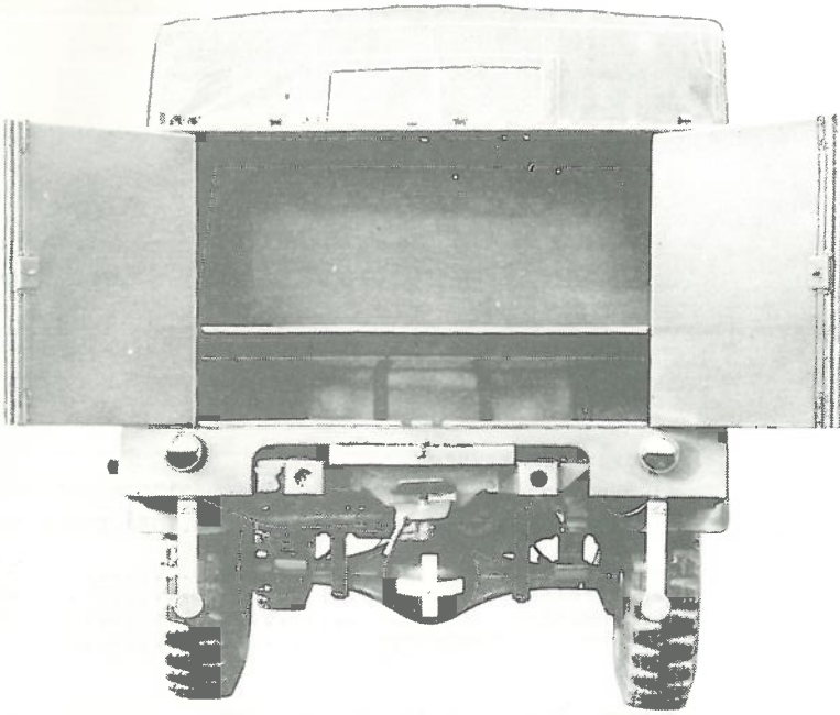
Hecktür des 0,75 t gl geöffnet mit Einbauteilen zur Einrichtung eines LKW als Fernsprechwagen
